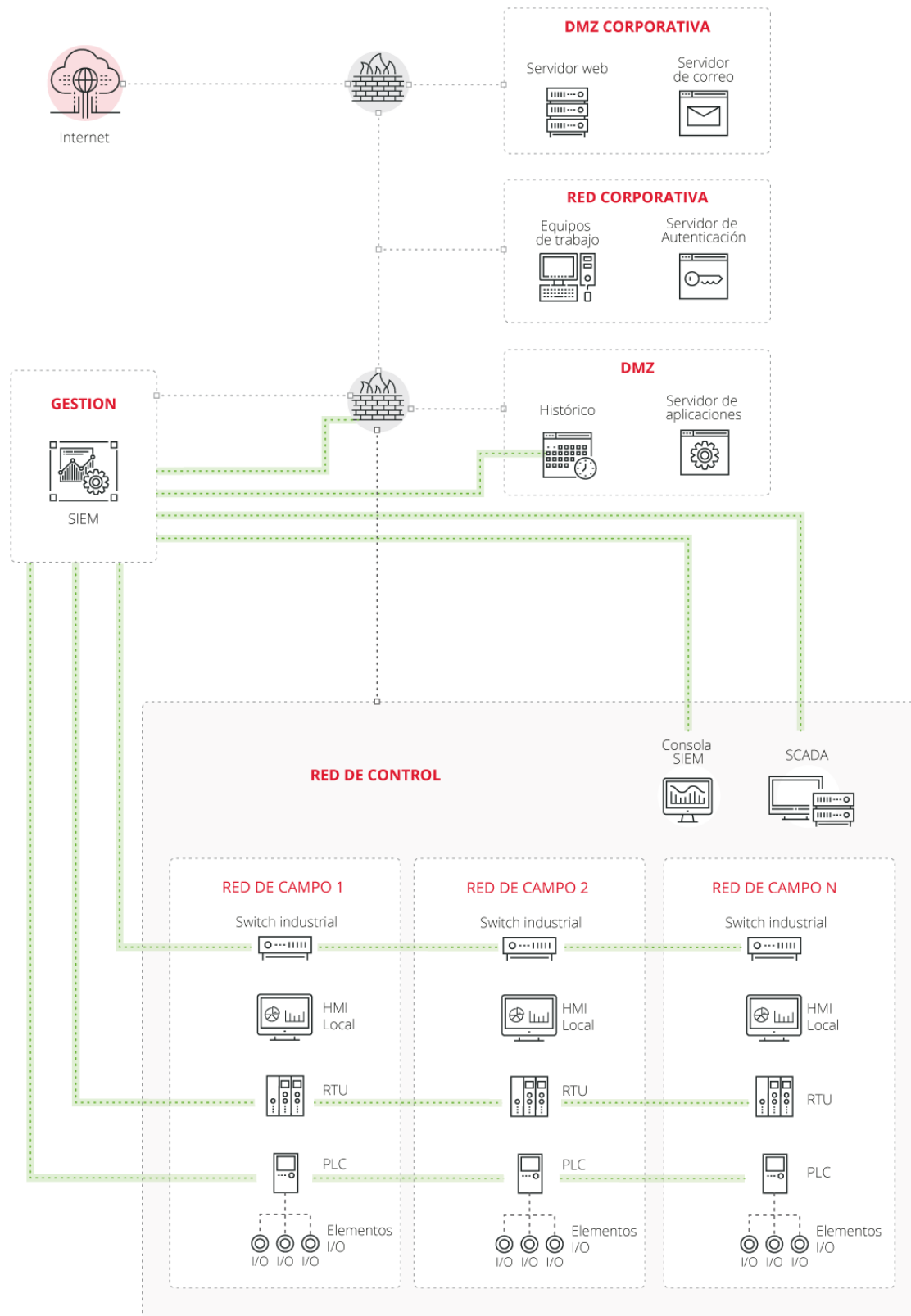
Figura 4: Arquitectura de seguridad con SIEM
