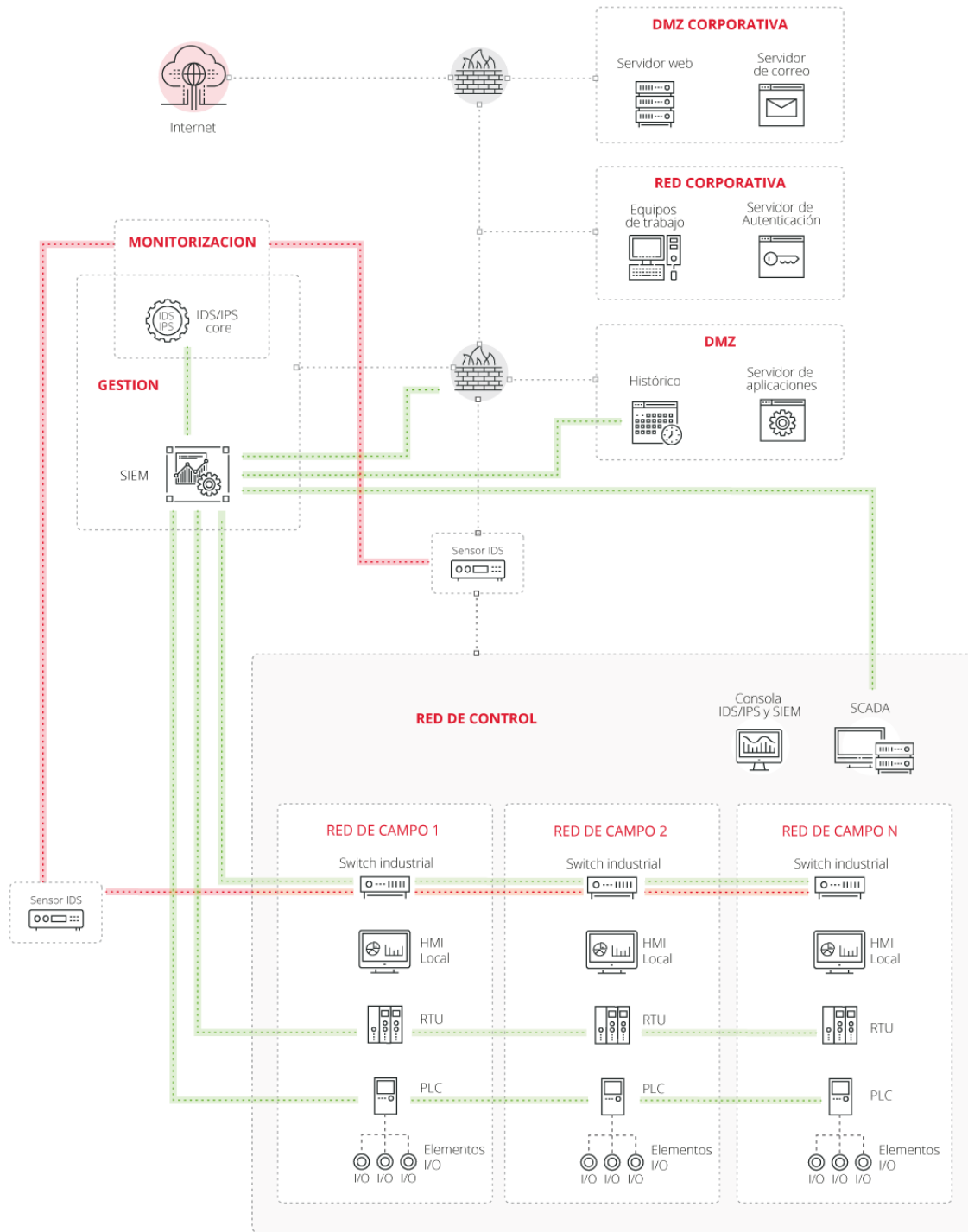
Figura 5: Arquitectura unificada con IDS, IPS y SIEM
