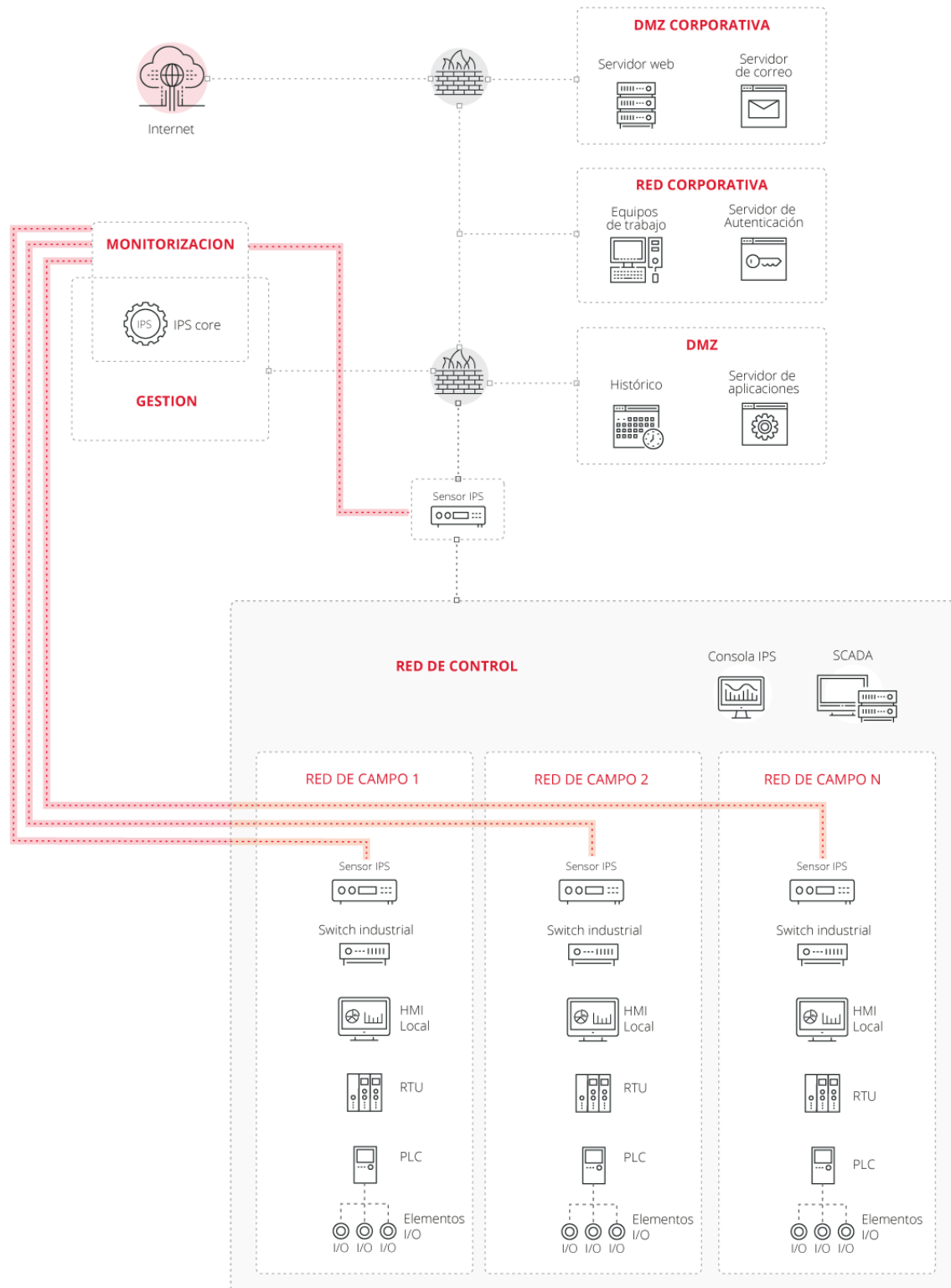
Figura 3: Arquitectura de seguridad con IPS
