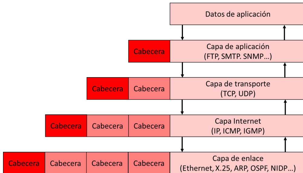
Figura 16: Encabezado y contenido de paquetes dependiendo del protocolo.
