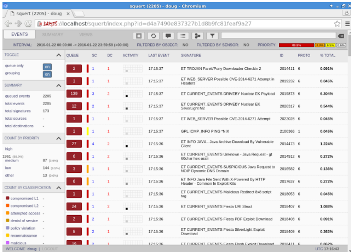
Figura 27: Cola de alertas en la pestaña de eventos de Squert 25
