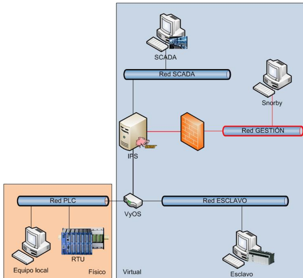
Figura 6: Arquitectura de despliegue en laboratorio
