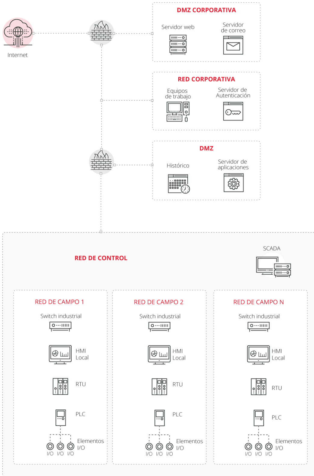
Figura 1: Arquitectura base para un sistema de control
