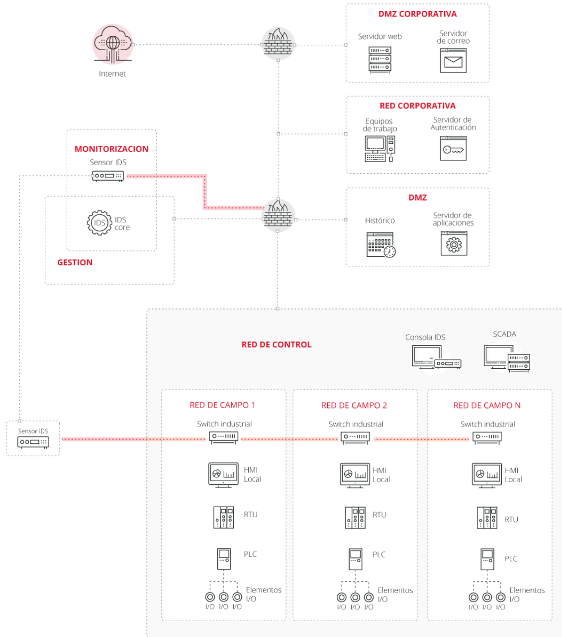
Figura 2: Arquitectura de seguridad con IDS
