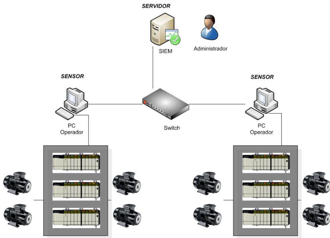
Figura 18: Ejemplo de SIEM en una red industrial
