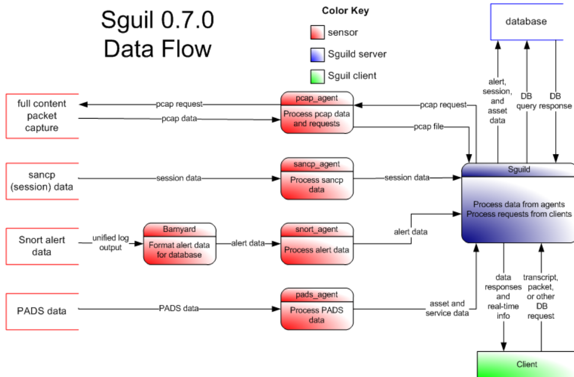
Figura 26: Flujo de datos de Sguil 24
