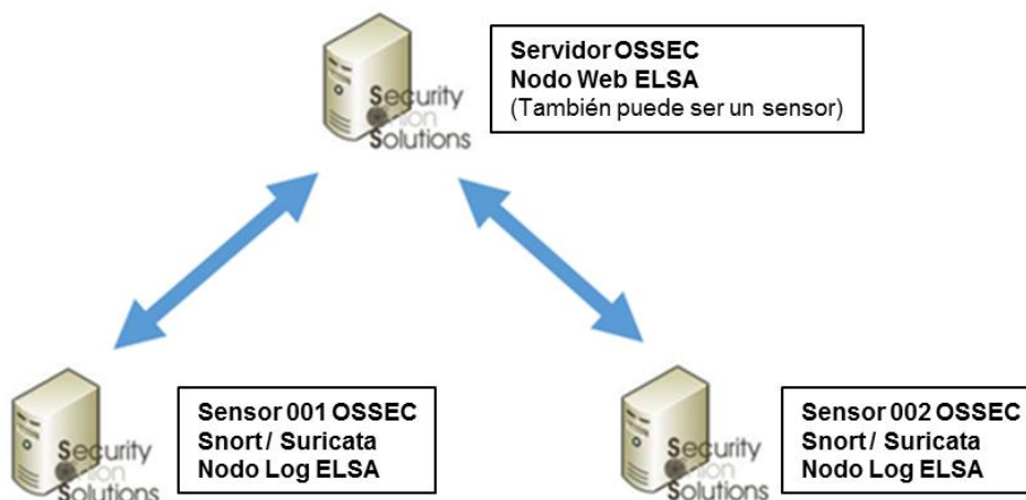
Figura 23: Arquitectura OSSEC
