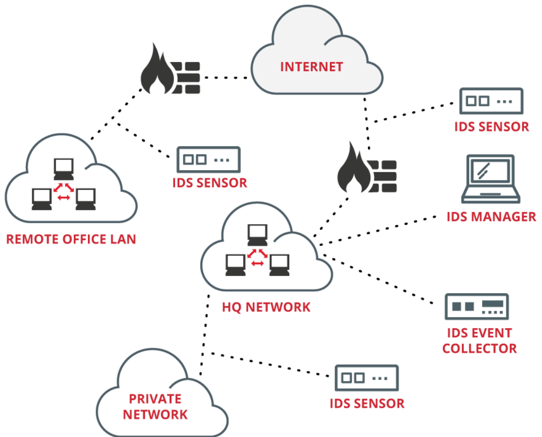
Figura 15: Ejemplo de IDS Centralizado. Fuente: Internet 4
